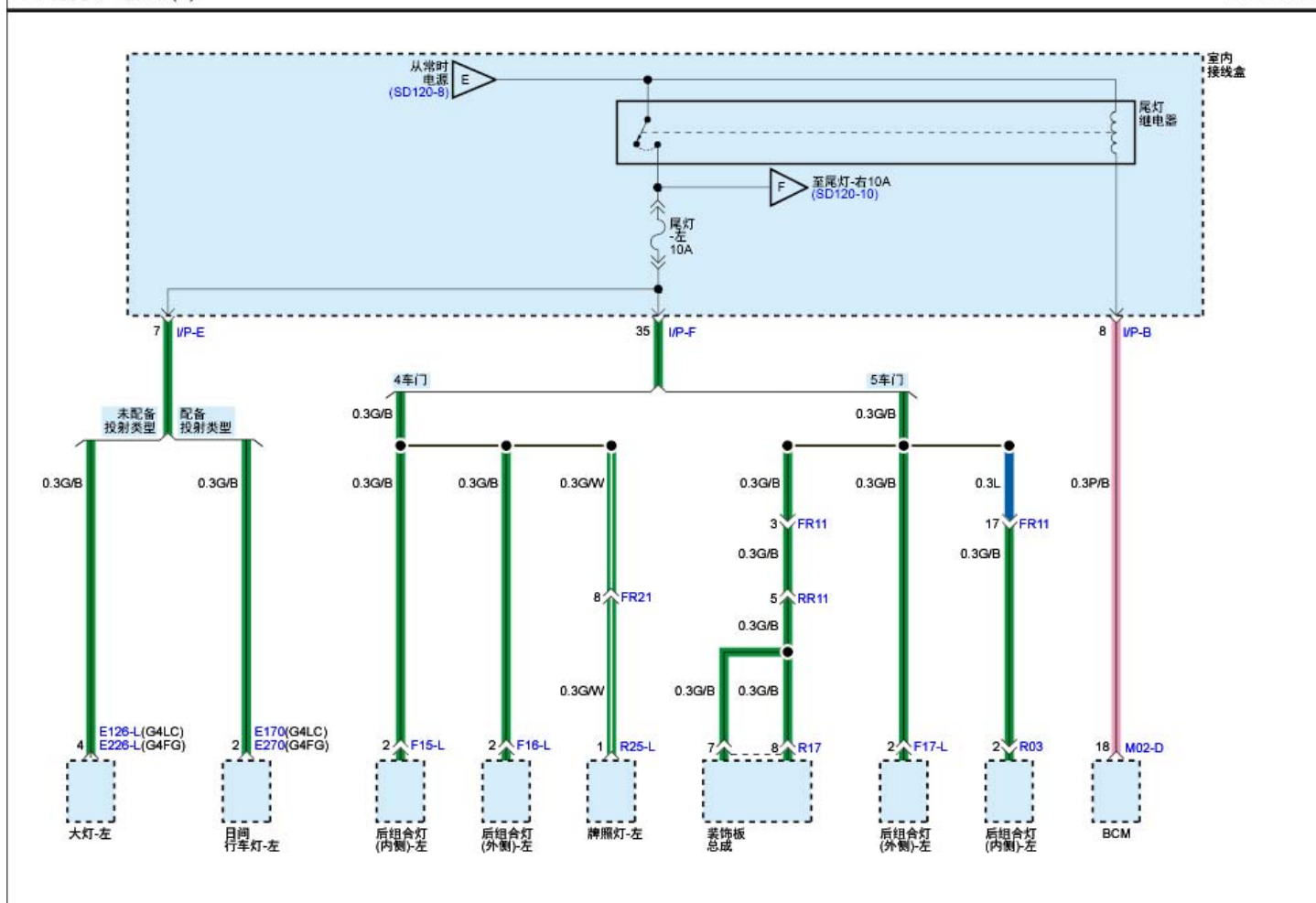
室内保险丝分布(9)
